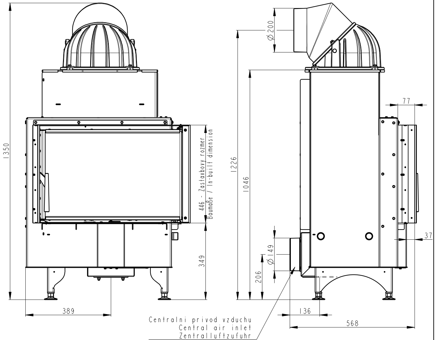
Otocna kopule s kolenom Cast iron turning dome Rotierende Kuppel mit Knie
